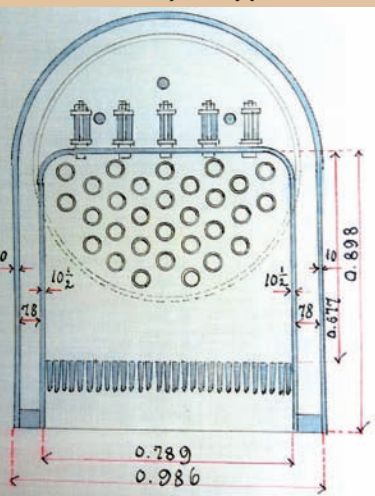
Poprzeczny przekrój kotła, który miał 30 płomieniówek
